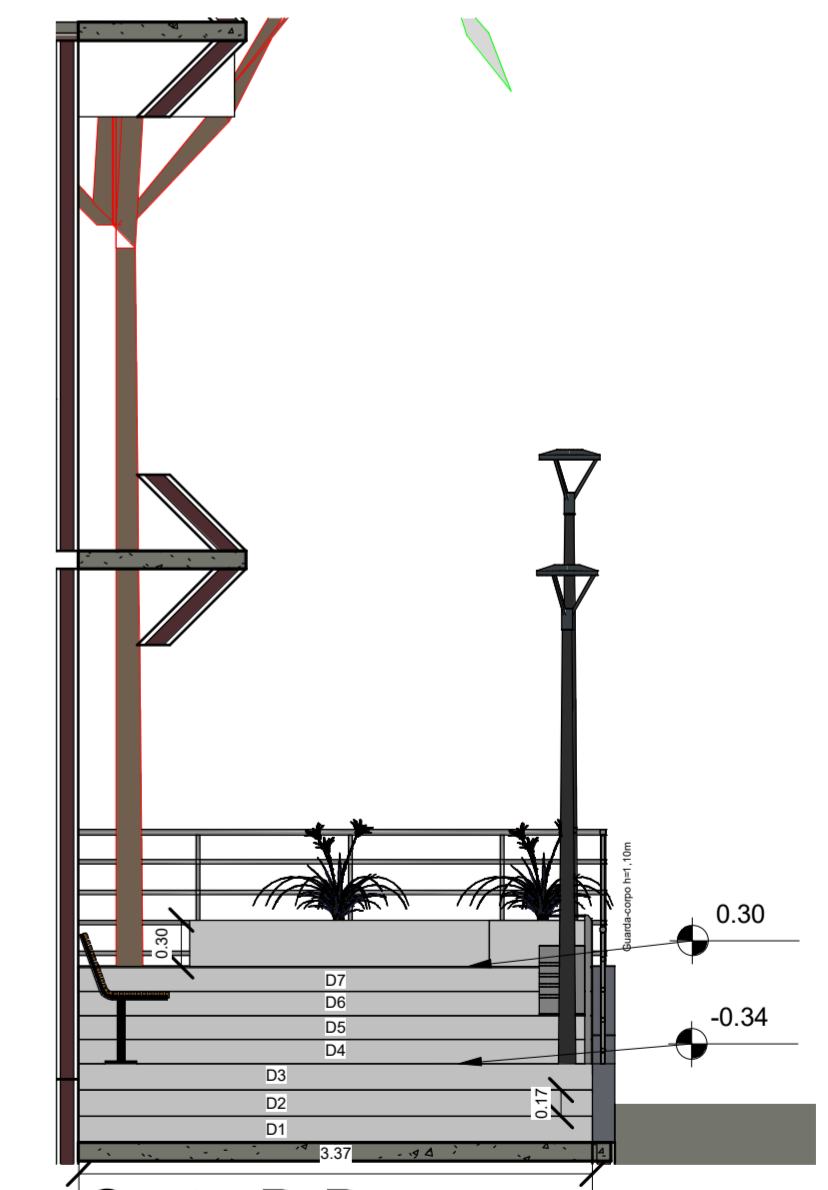
4 Corte B-B 1 : 50
