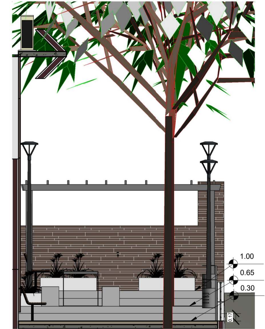
3 Corte A-A 1 : 50
