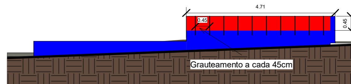
2 Muro av. sete de setembro 1 : 75
