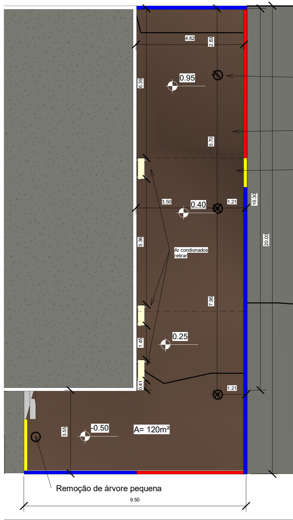
1 Planta existente 1 : 100
