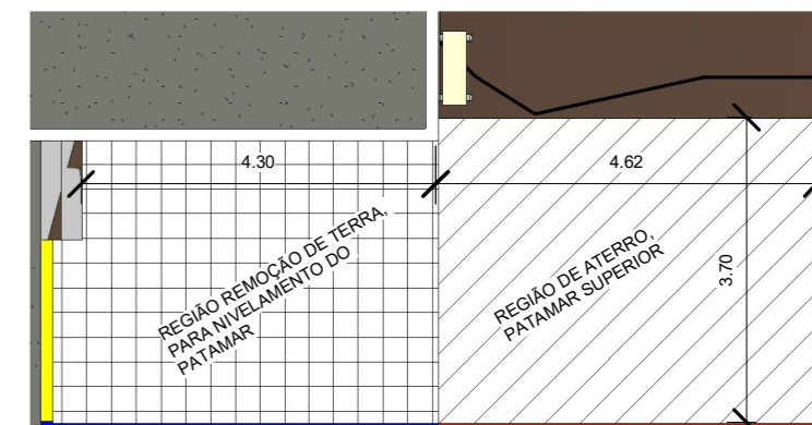
5 Planta aterro 1 : 100
