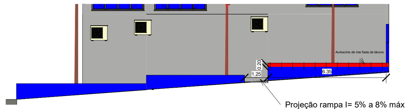
3 Muro rua bandeirantes 1 : 125
