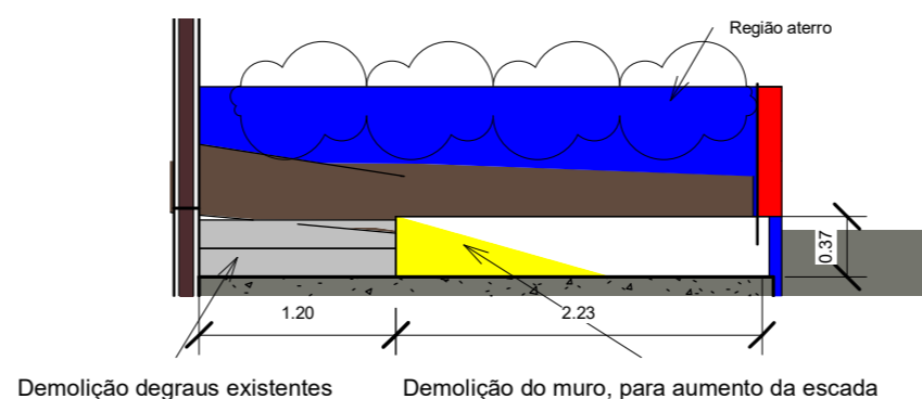
4 Muro interno - escada 1 : 50
